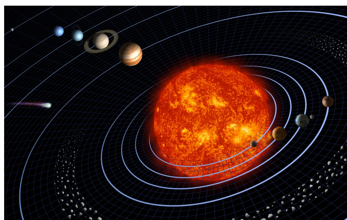
il Sistema solare: al centro c'è il Sole
