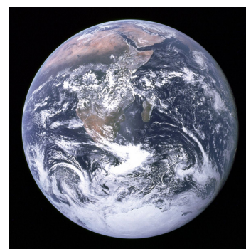
la Terra vista dallo spazio
